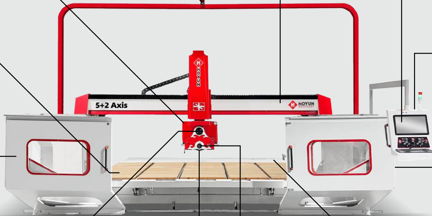
Camera 相机
